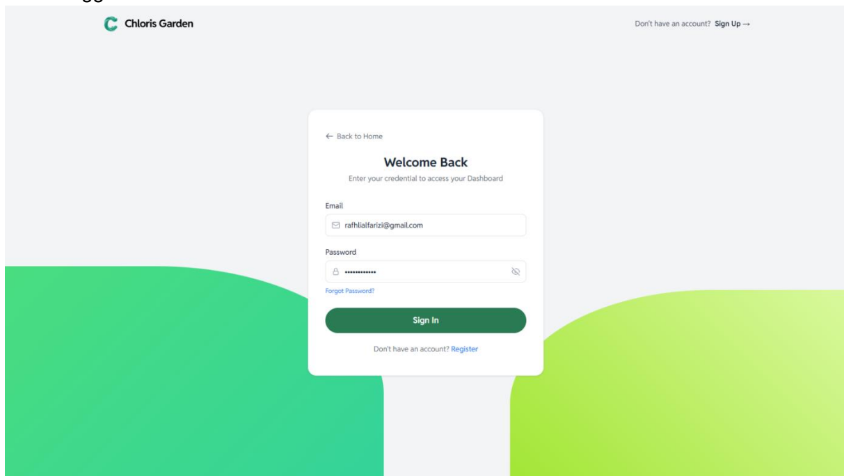
Gambar 3 Halaman Login
